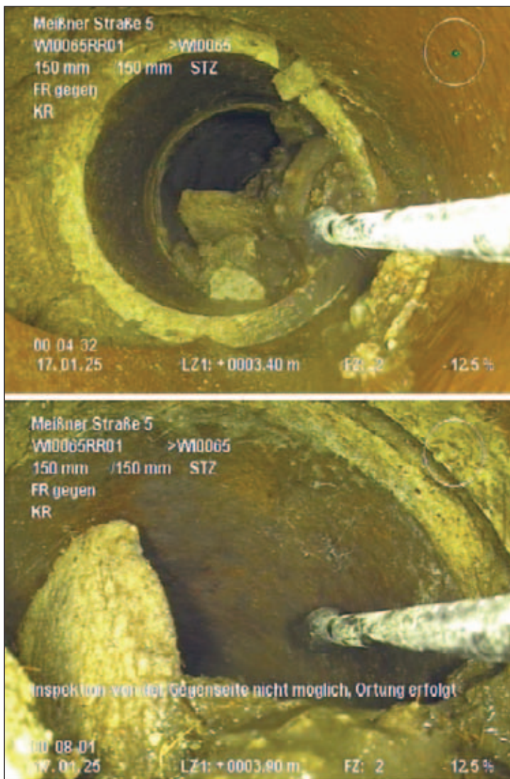
defekter Anschlusskanal in der Meißner Straße
